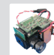
車載用プロジェクター
